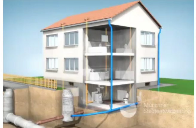
Querschnitt Abwasserleitungen
