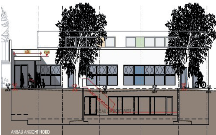
Schematischer Schnitt der Nordansicht des Erd- und Kellergeschosses des neuen Kinderbetreuungscomplexes
