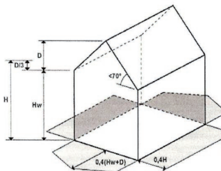
Berechnungsbeispiel für die neuen Abstandsflächen der BayBO
