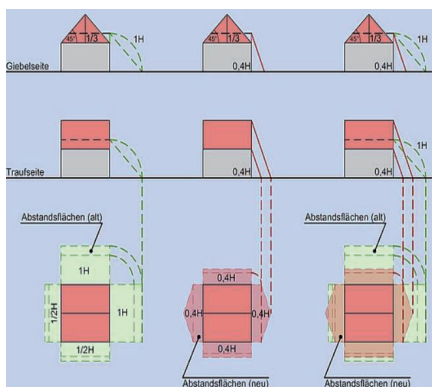
Schematische Darstellung für einen groben Überblick im Wirrwarr der neuen Abstandsregelungen
